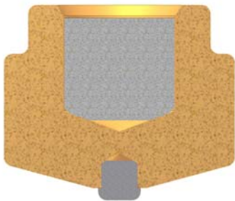
Abb 2.: Schnittzeichnung und Foto TungStud (Quelle: BETEK)
